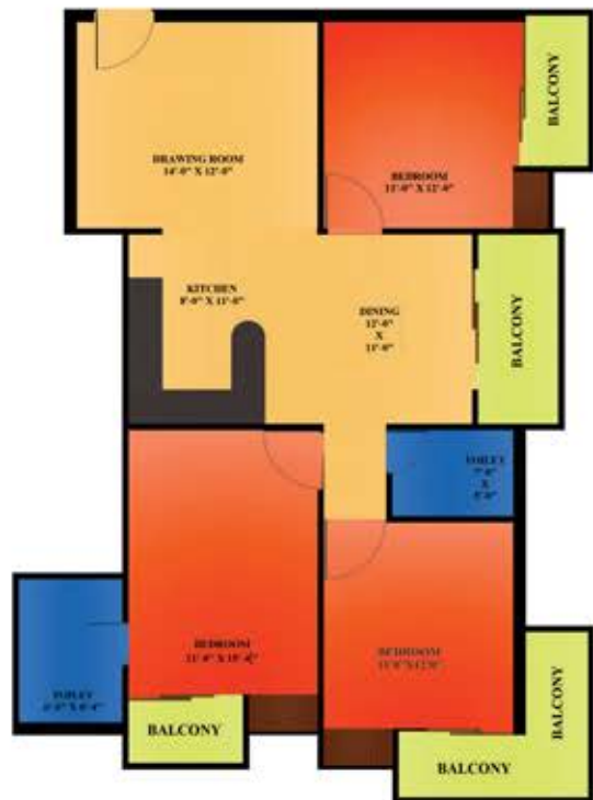
3BHK Type 2 PLAN -
